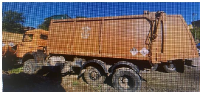
Фото 5. Транспортное средство машина коммунальная КО-440-5 мусоровоз, 2007 года
