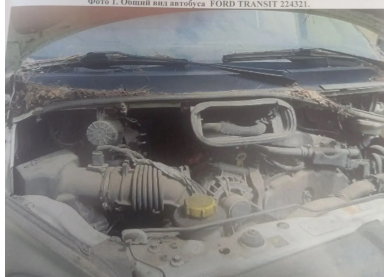
Фото 1. Общий вид автобуса FORD TRANSIT 224321
